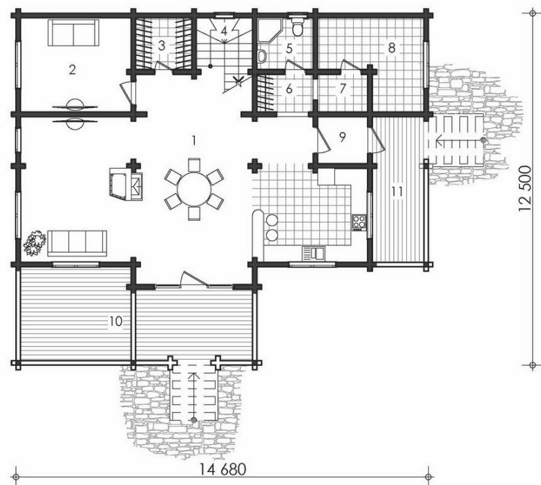
План первого этажа
