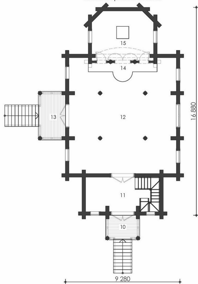
План первого этажа
